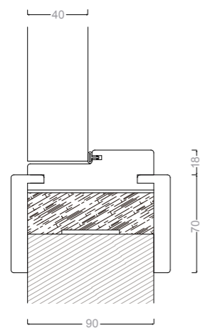
Detalle en sección del cerco
