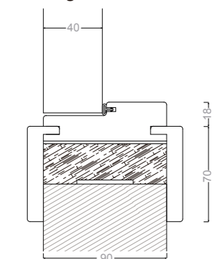
Detalle en sección de la guía
