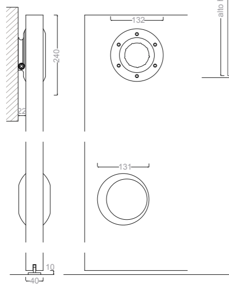
Detalle en sección de la guía
