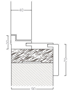
Detalle en sección del cerco
