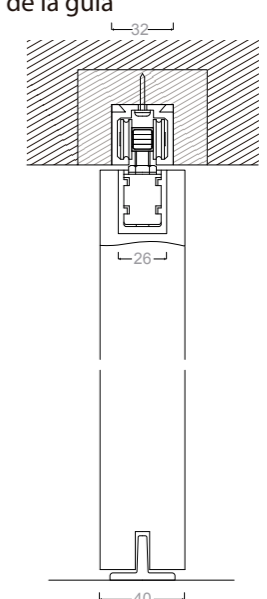
Detalle en sección de la guía
