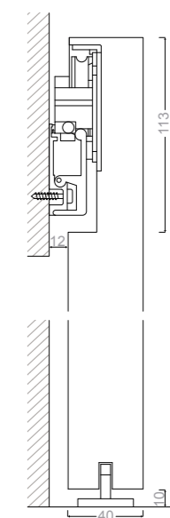
Detalle en sección de la guía
